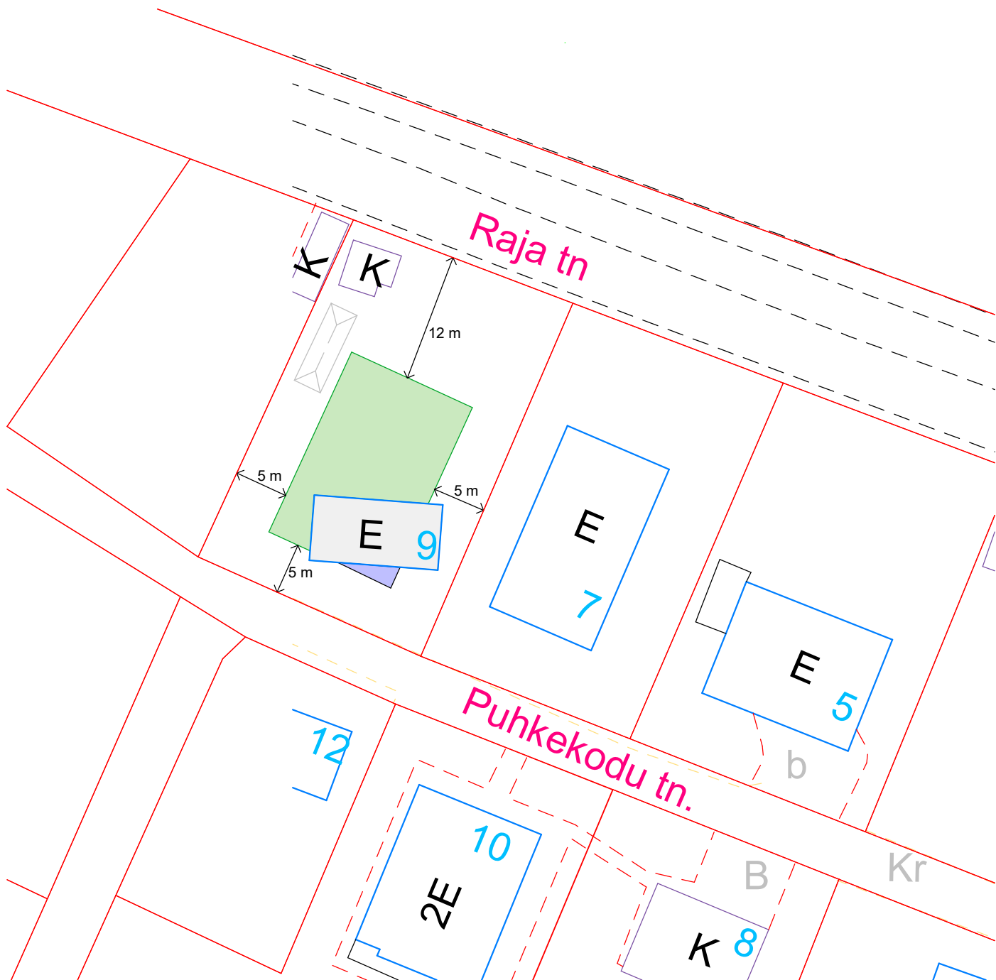
Lisa. Puhkekodu tn 9 ehitusala skeem PTH-22-086
